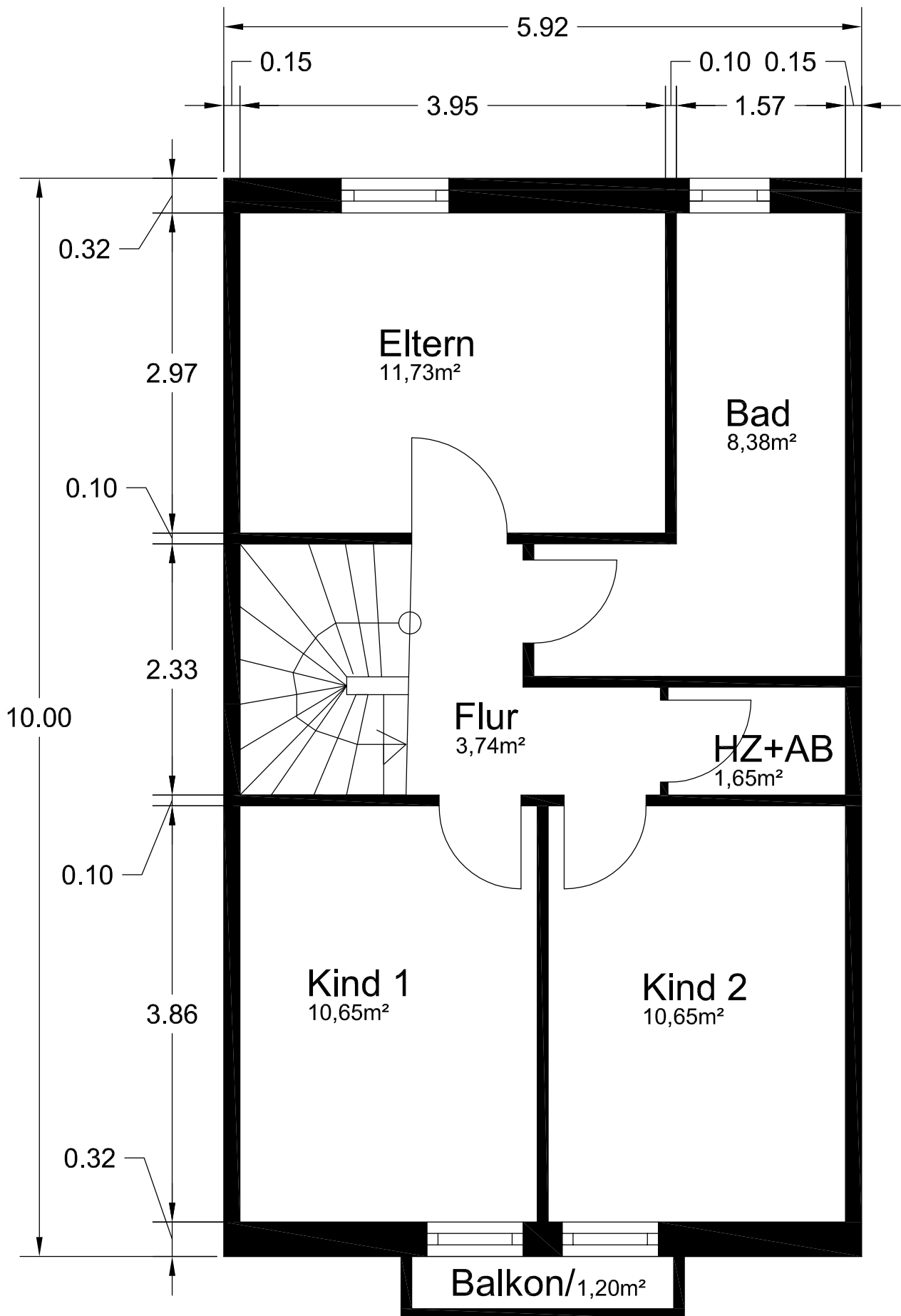
Obergeschoss: Beispiel Grundriss - Individuell Anpassbar
