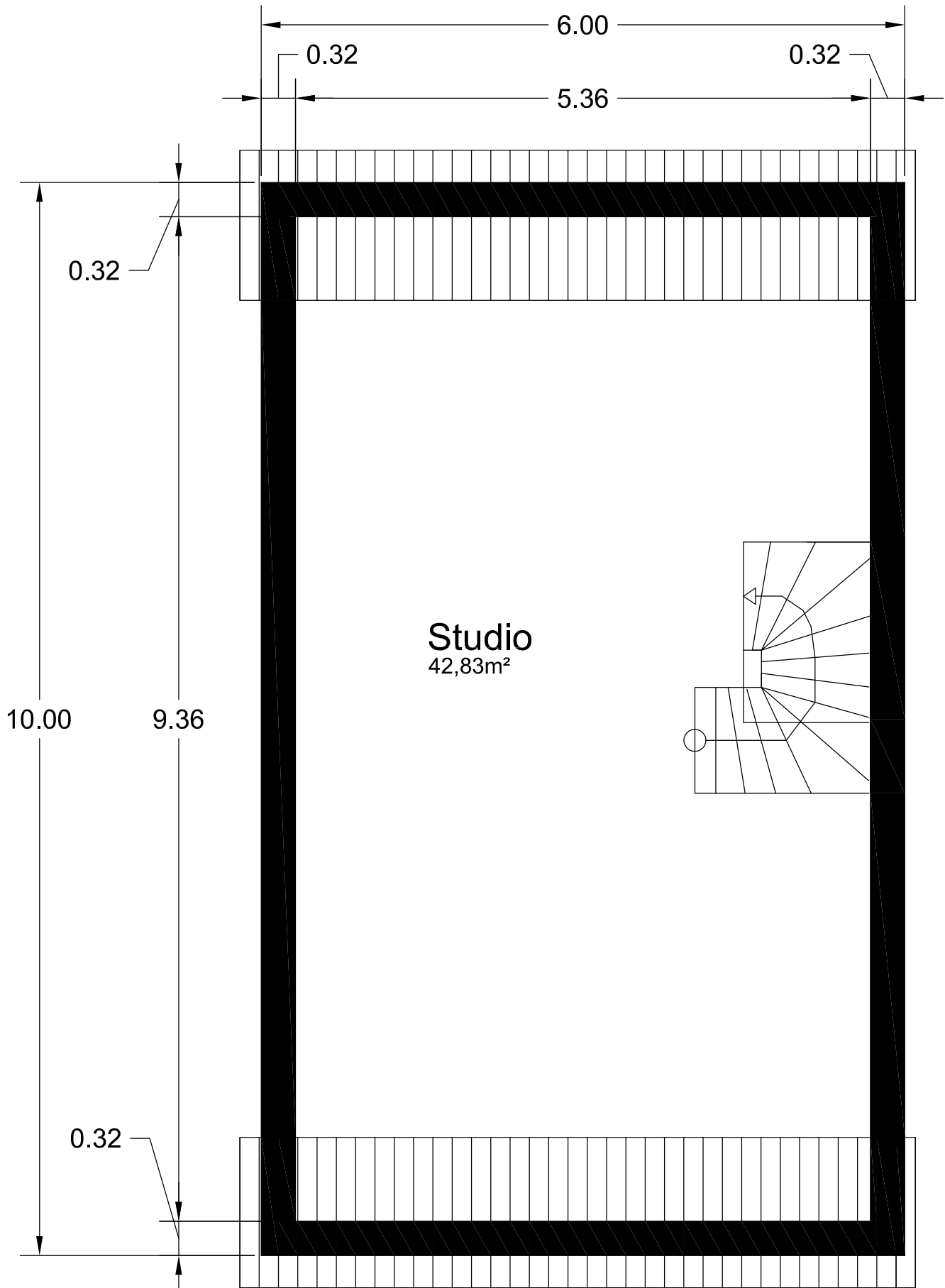
Dachgeschoss: Beispiel Grundriss - Individuell Anpassbar
