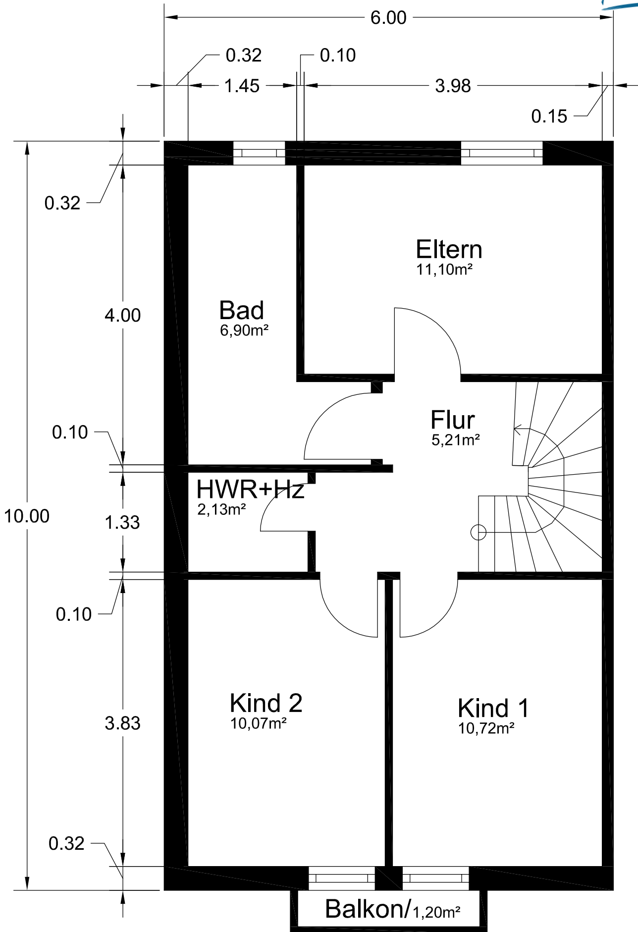
Obergeschoss: Beispiel Grundriss - Individuell Anpassbar
